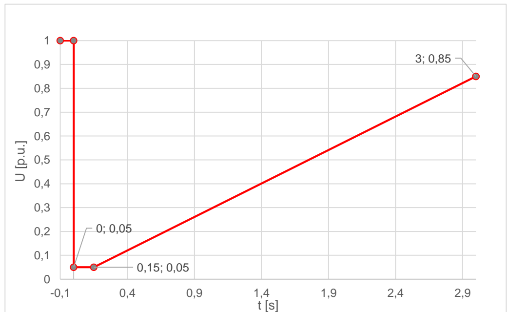
Obr. 5 Časovým průběhem napětí v místě připojení za podmínek poruchy pro nesynchronní výrobní moduly kategorie A1, A2, B1, B2 a C (FRT křivka)
