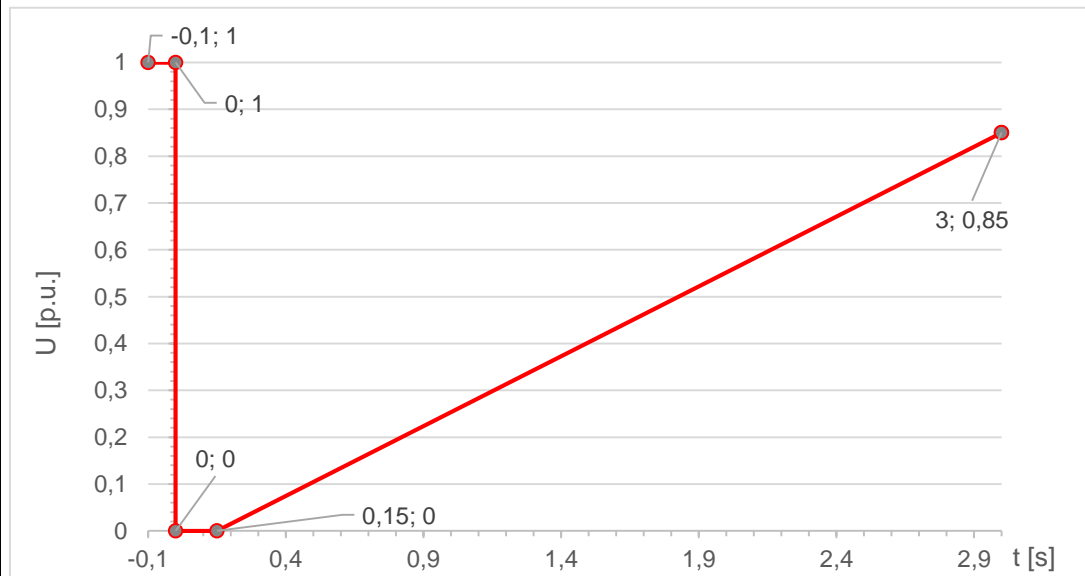
Obr. 8 Časovým průběhem napětí v místě připojení za podmínek poruchy pro nesynchronní výrobní moduly kategorie D (FRT křivka)
